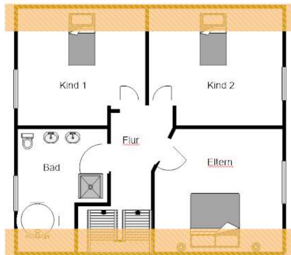
3 von 3 Grundriss DG
