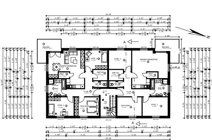
GRUNDRISS OBERGESCHOSS
