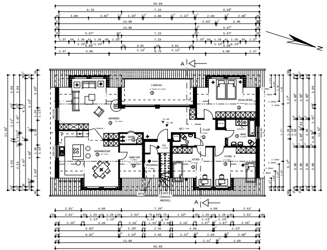
GRUNDRISS DACHGESCHOSS
