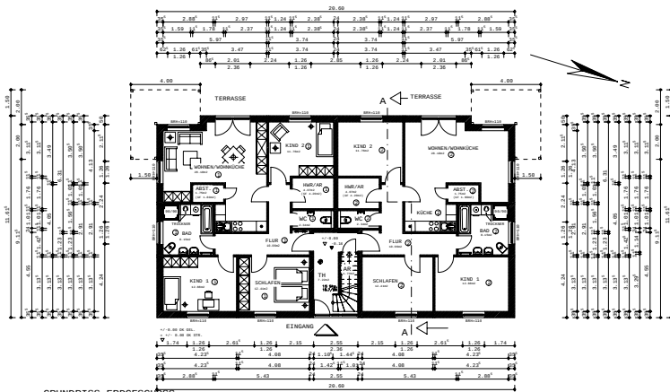
GRUNDRISS ERDGESCHOSS
