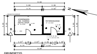
GRUNDRISS
