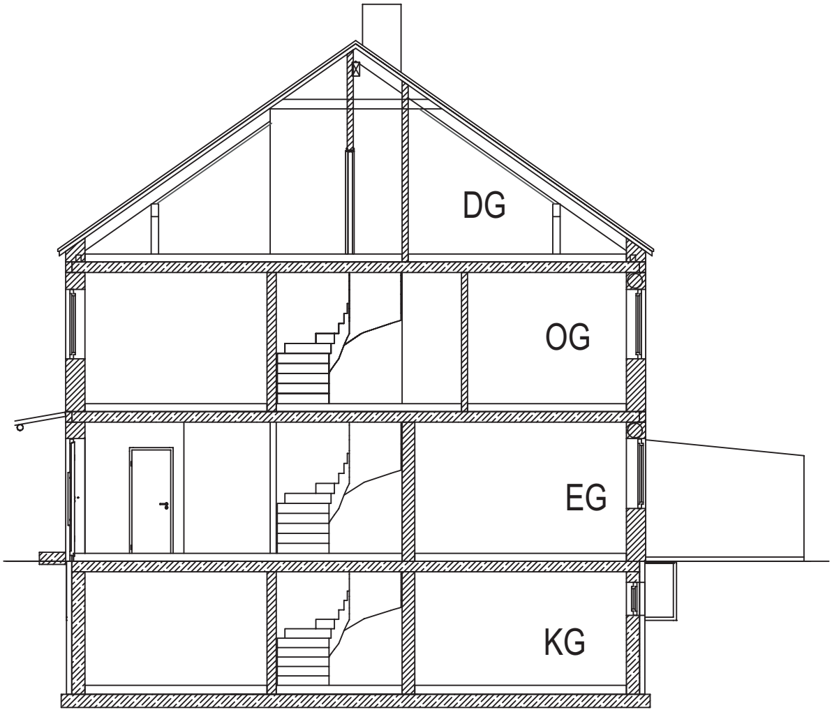
Schnitt
