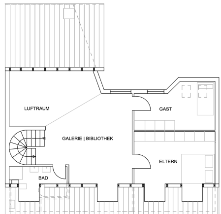
GRUNDRISS DG
