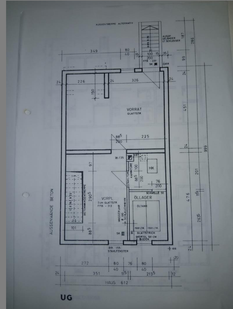
Grundriss UG
