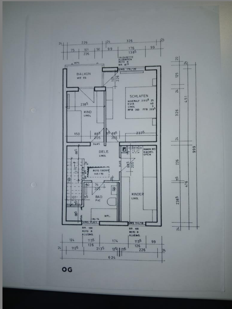
Grundriss 1. OG
