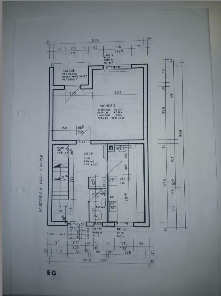
EG vor Wintergartenerweiterung
