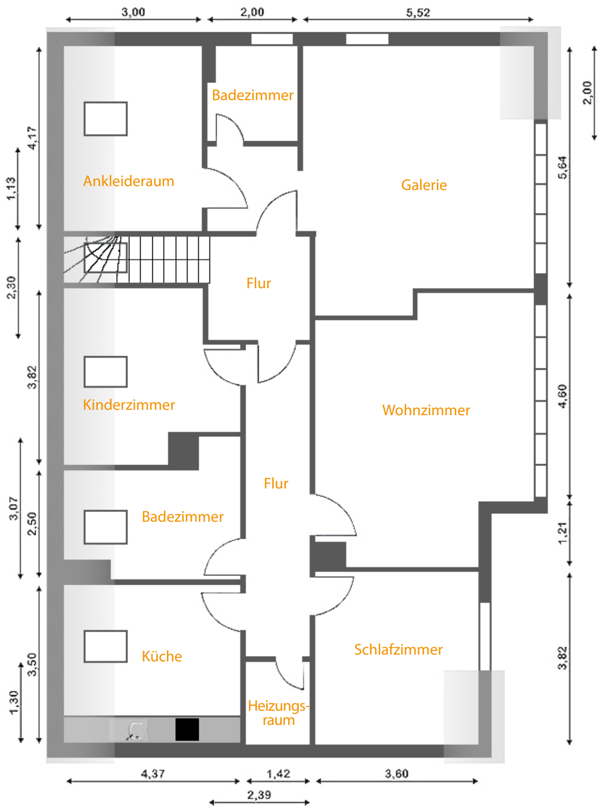
GRUNDRISS DACHGESCHOSS
