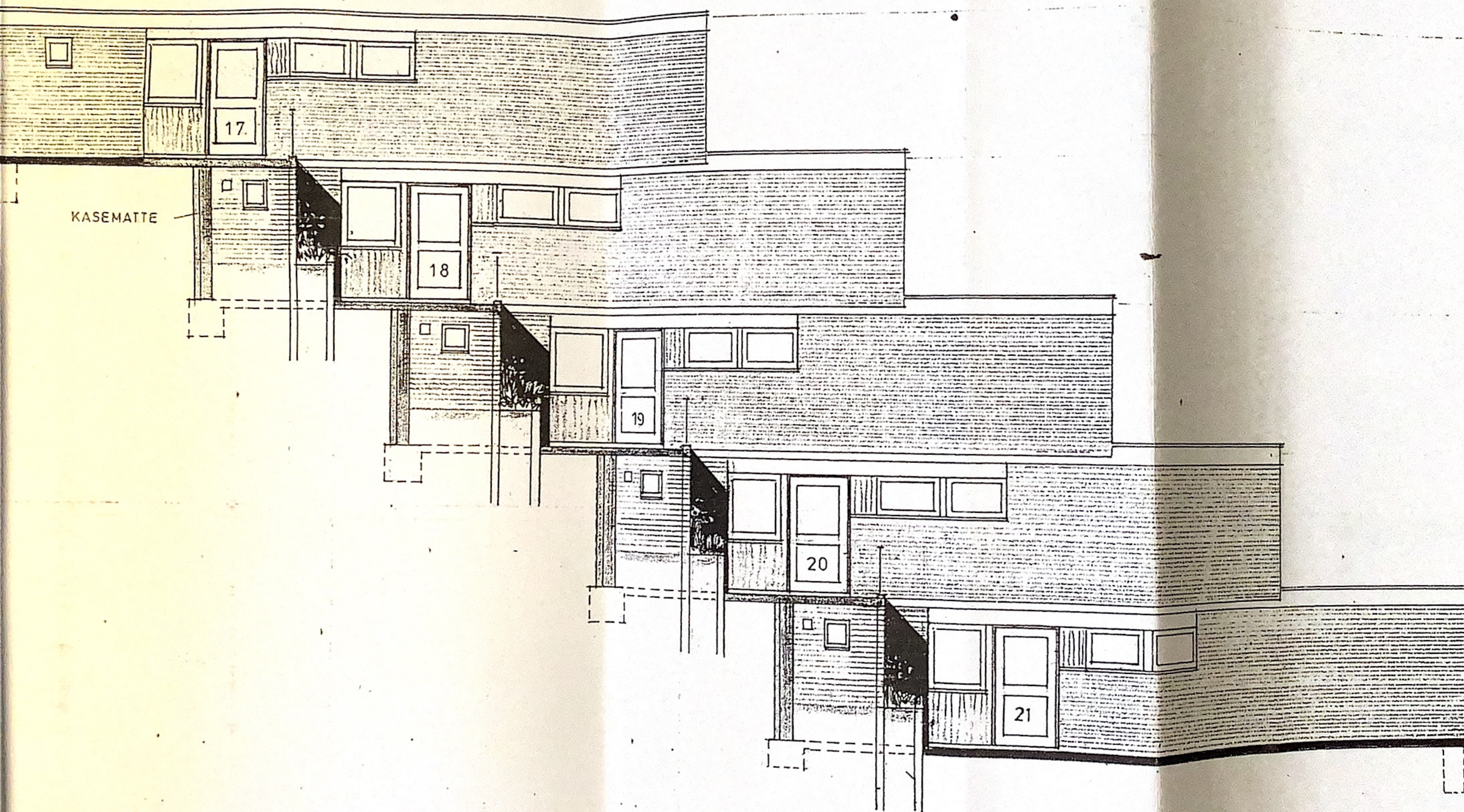
NORD - ANSICHT
