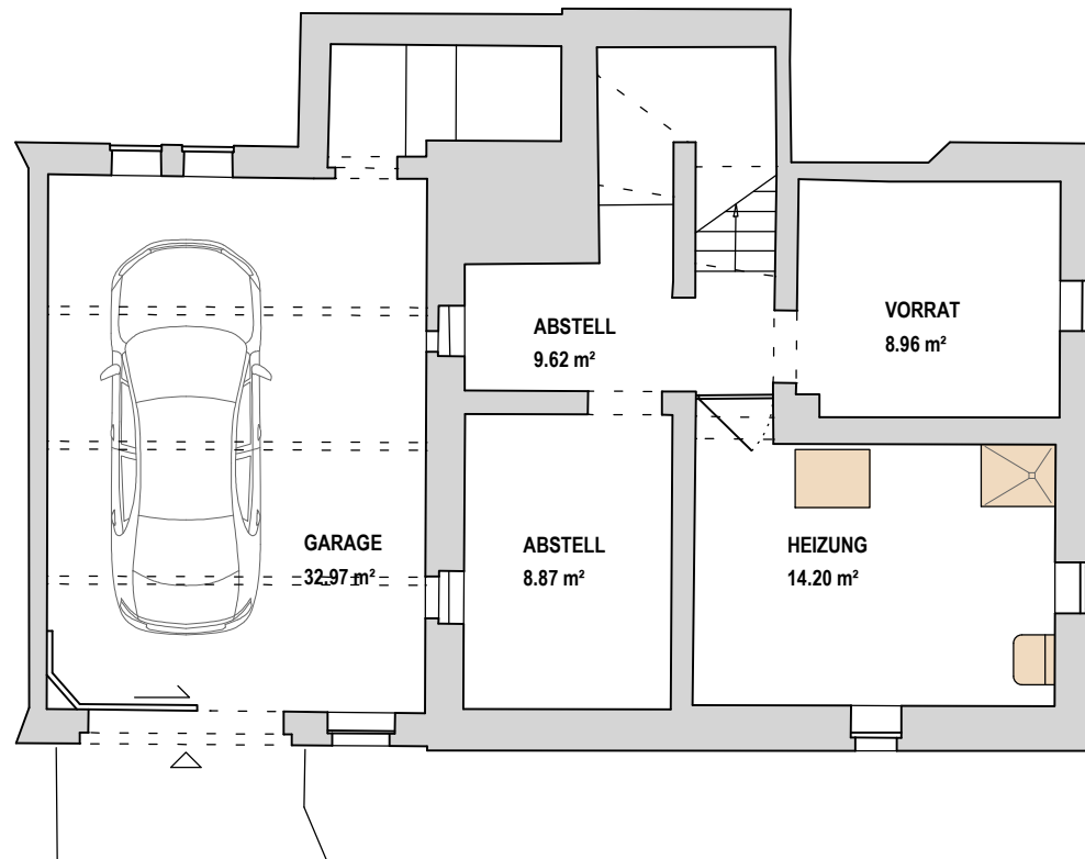
KELLERGESCHOSS
