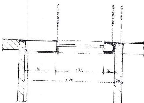
FENSTER SCHNITT 1:20
