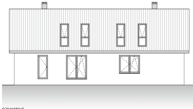
SÜDANSICHT
