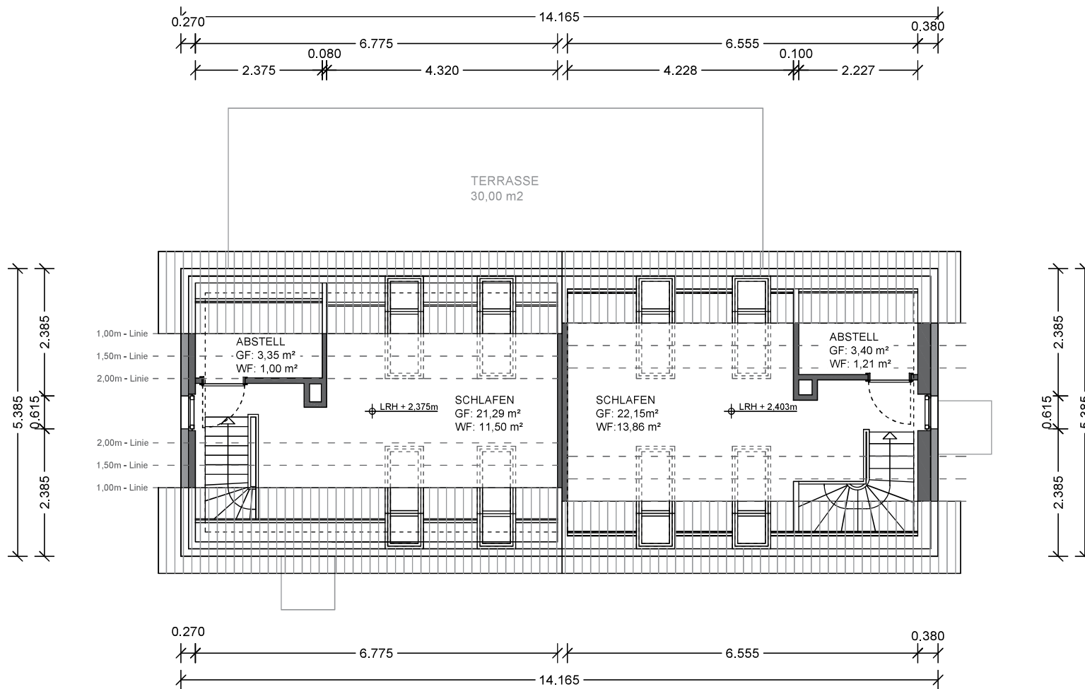
DACHGESCHOSS
