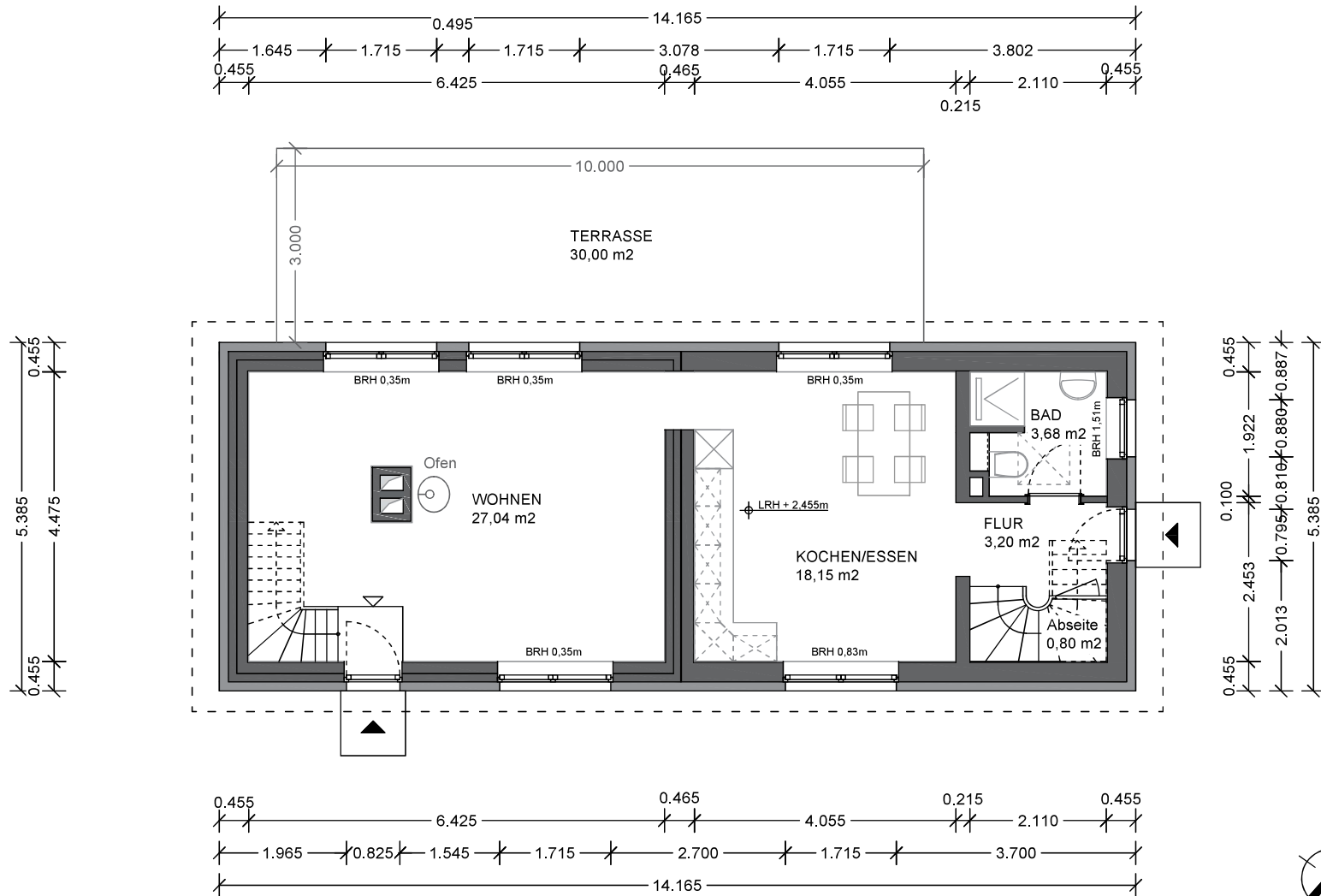
ERDGESCHOSS
