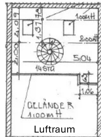
Grundriss oben: Maisonette
