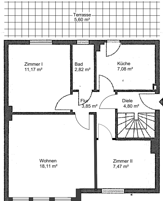
Grundriss Erdgeschoss
