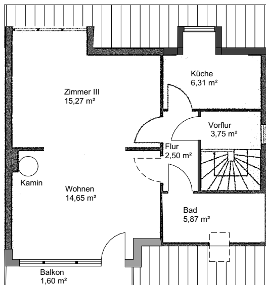
Grundriss Obergeschoss
