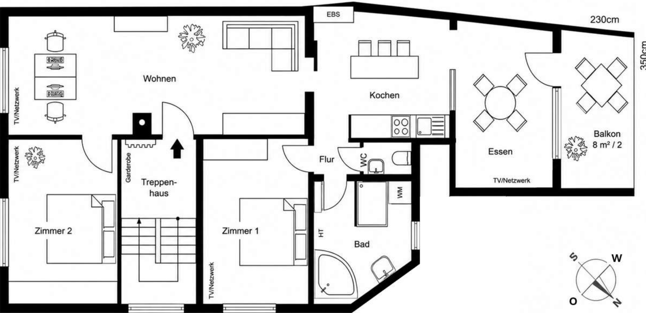
Obergeschoss
