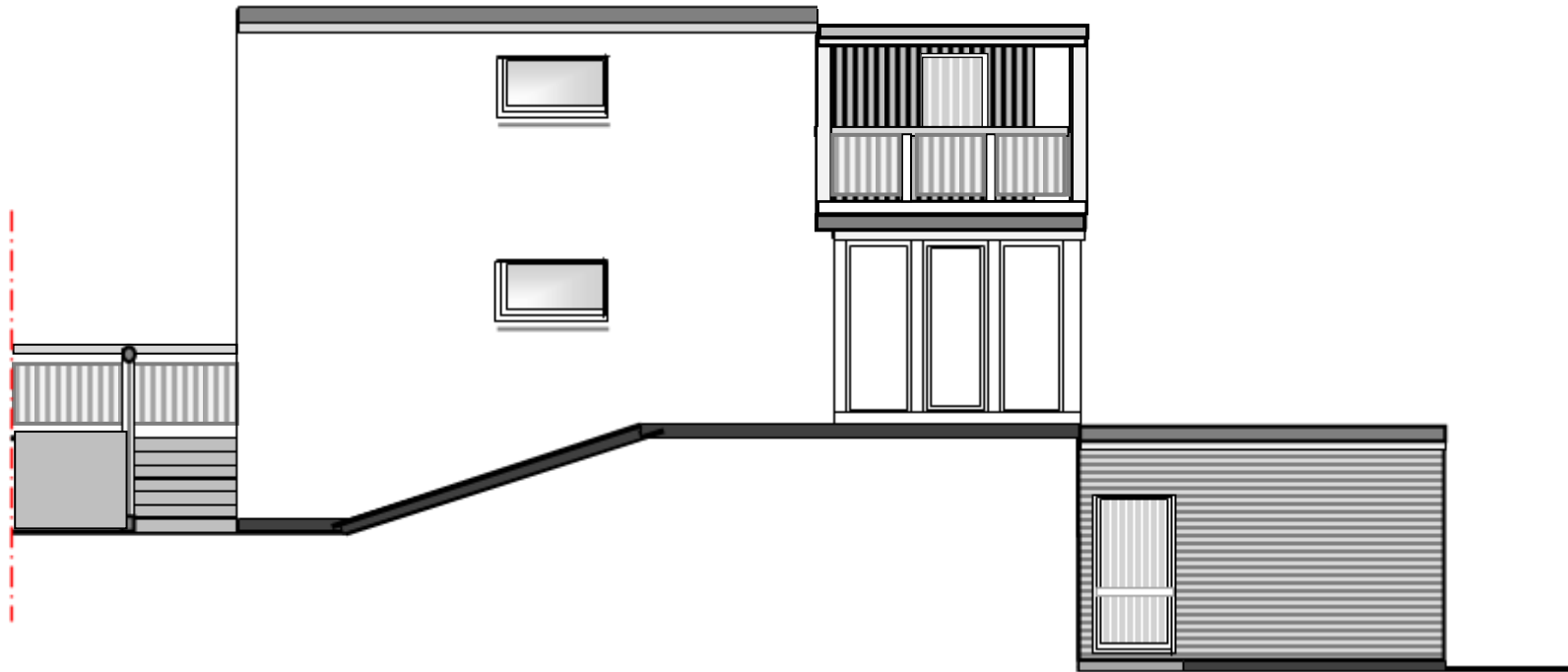
NORD-OST-ANSICHT
