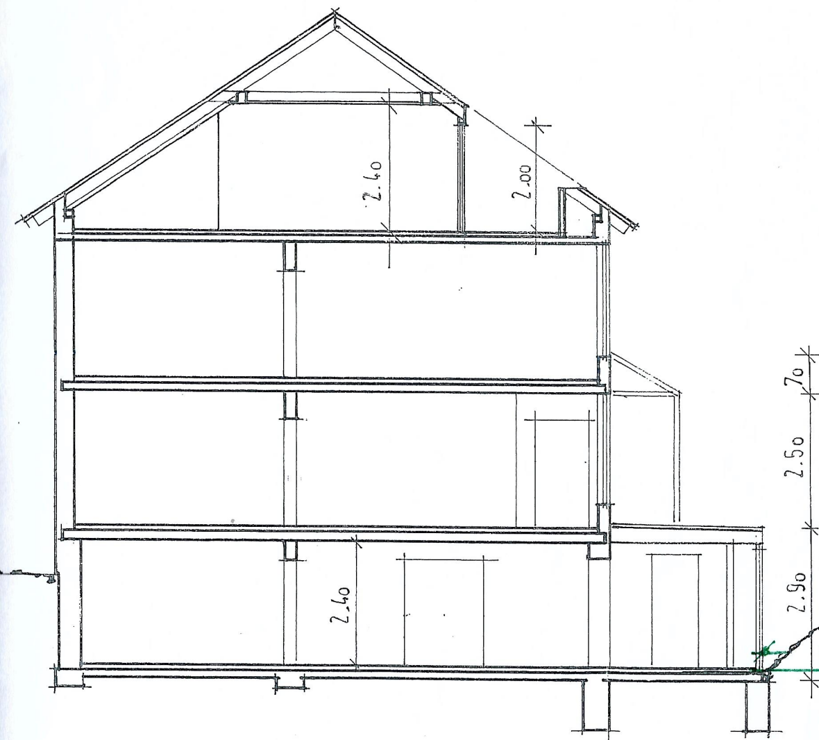
schnitt
