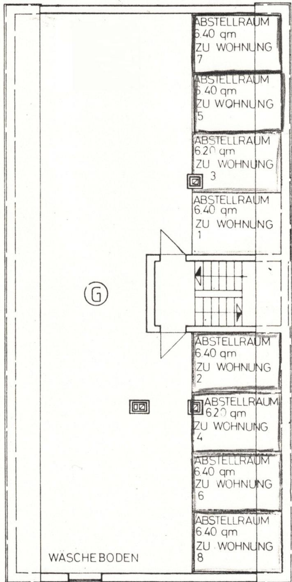
DACHGESCHOSS
