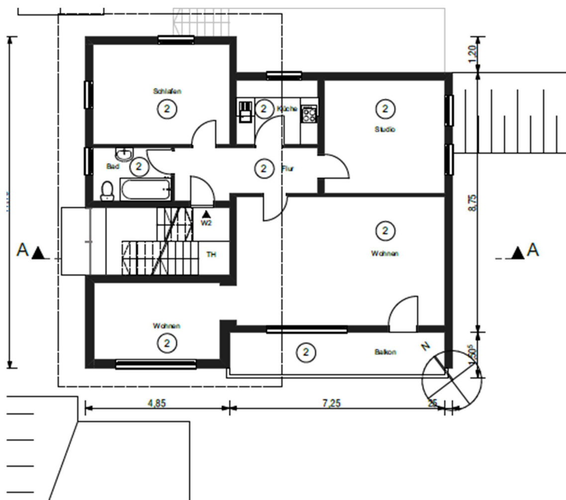
GRUNDRISS OBERGESCHOSS
