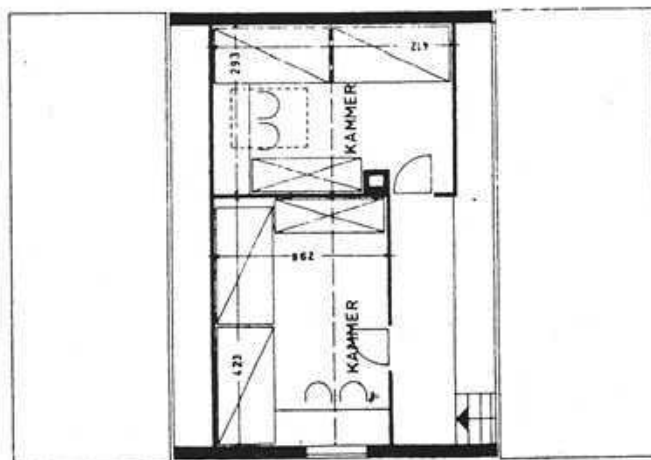
dachgeschoss ausbaumöglichkeit
