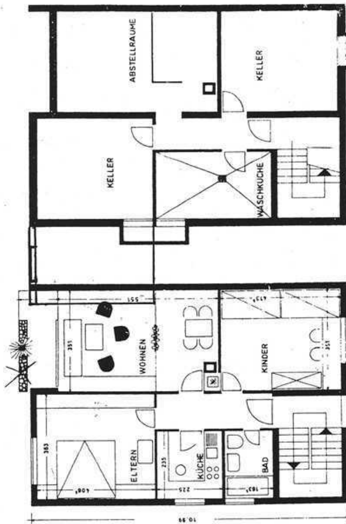
untergeschoss
