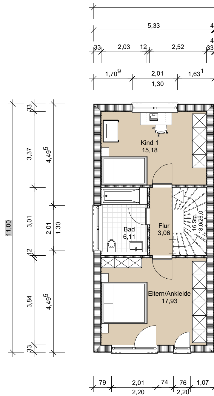
Haus West 1. OBERGESCHOSS
