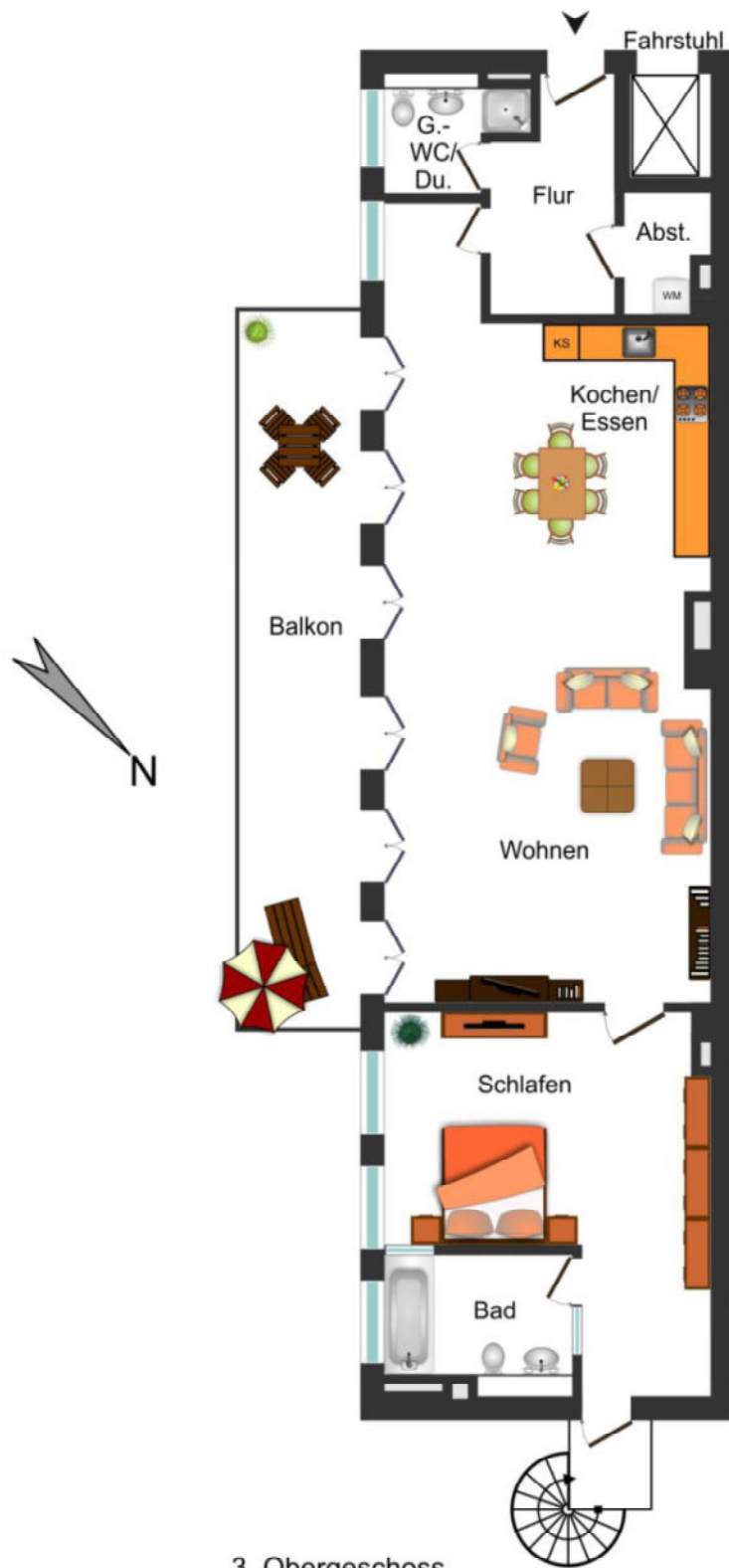
3. Obergeschoss
