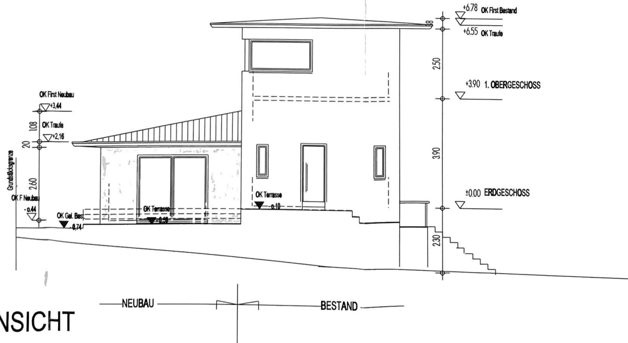
NORD-WESTANSICHT
