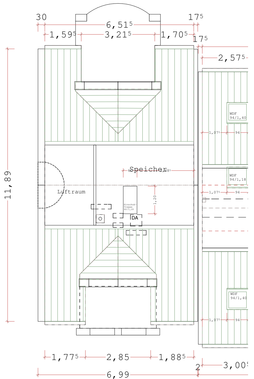
DACHAUFSICHT
