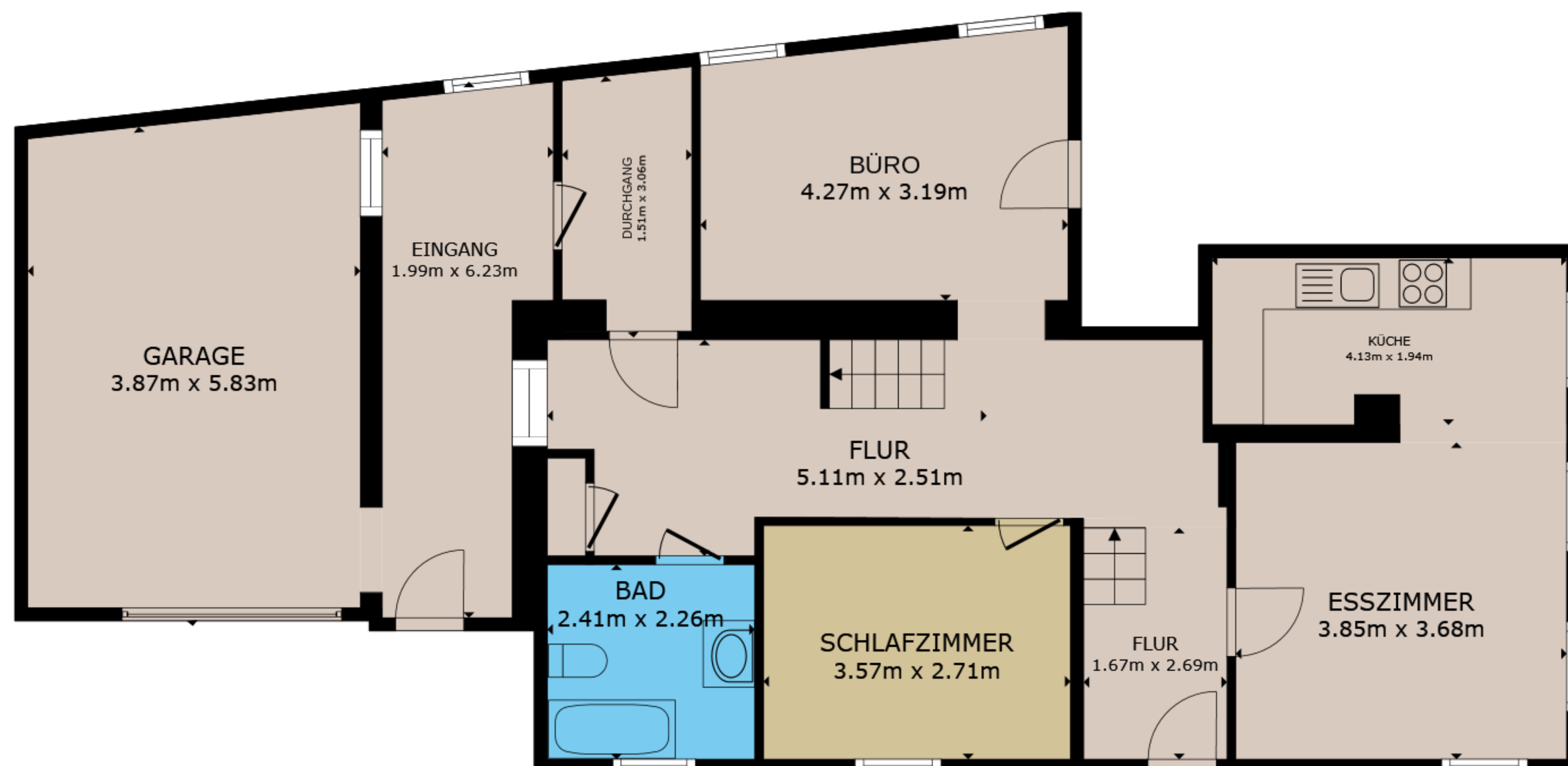
STOCKWERK 1
