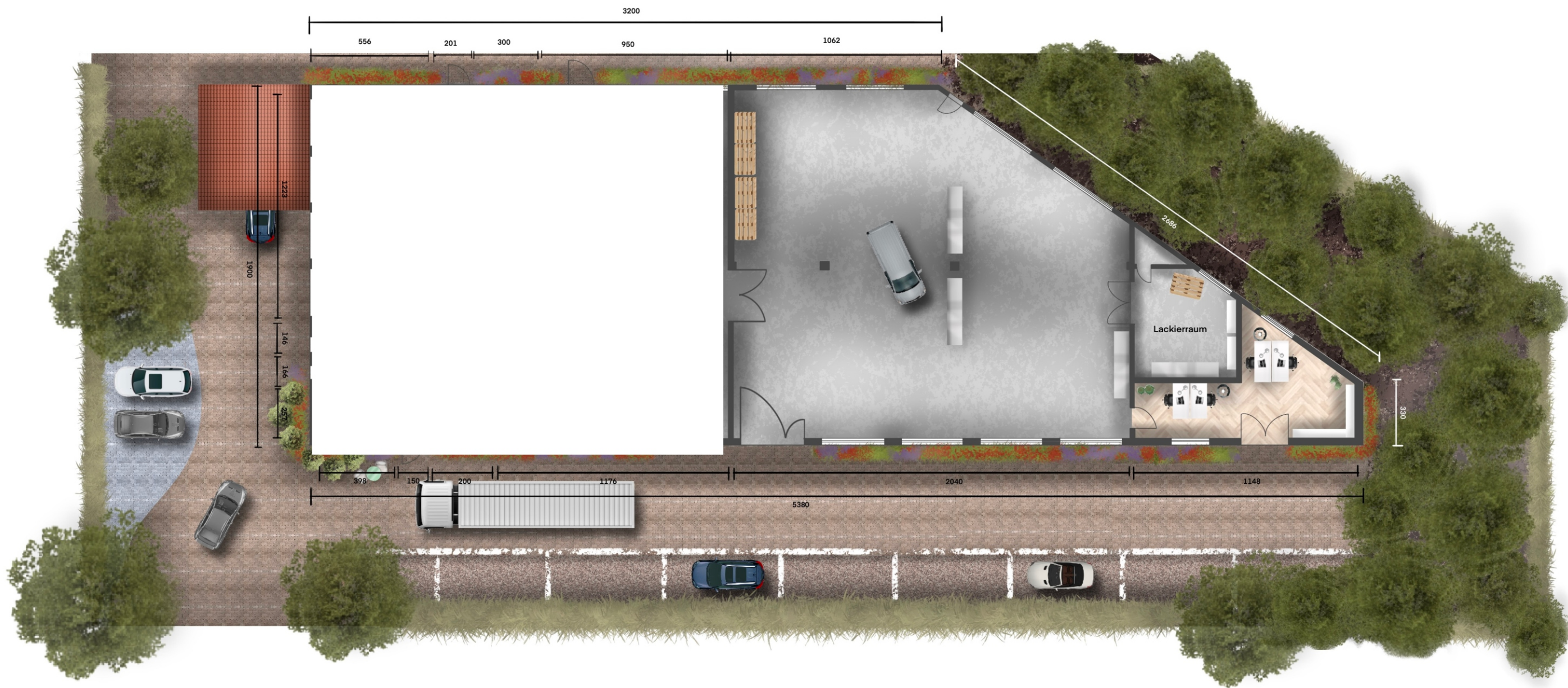
Grundriss EG MASSEINHEITEN IN CM
