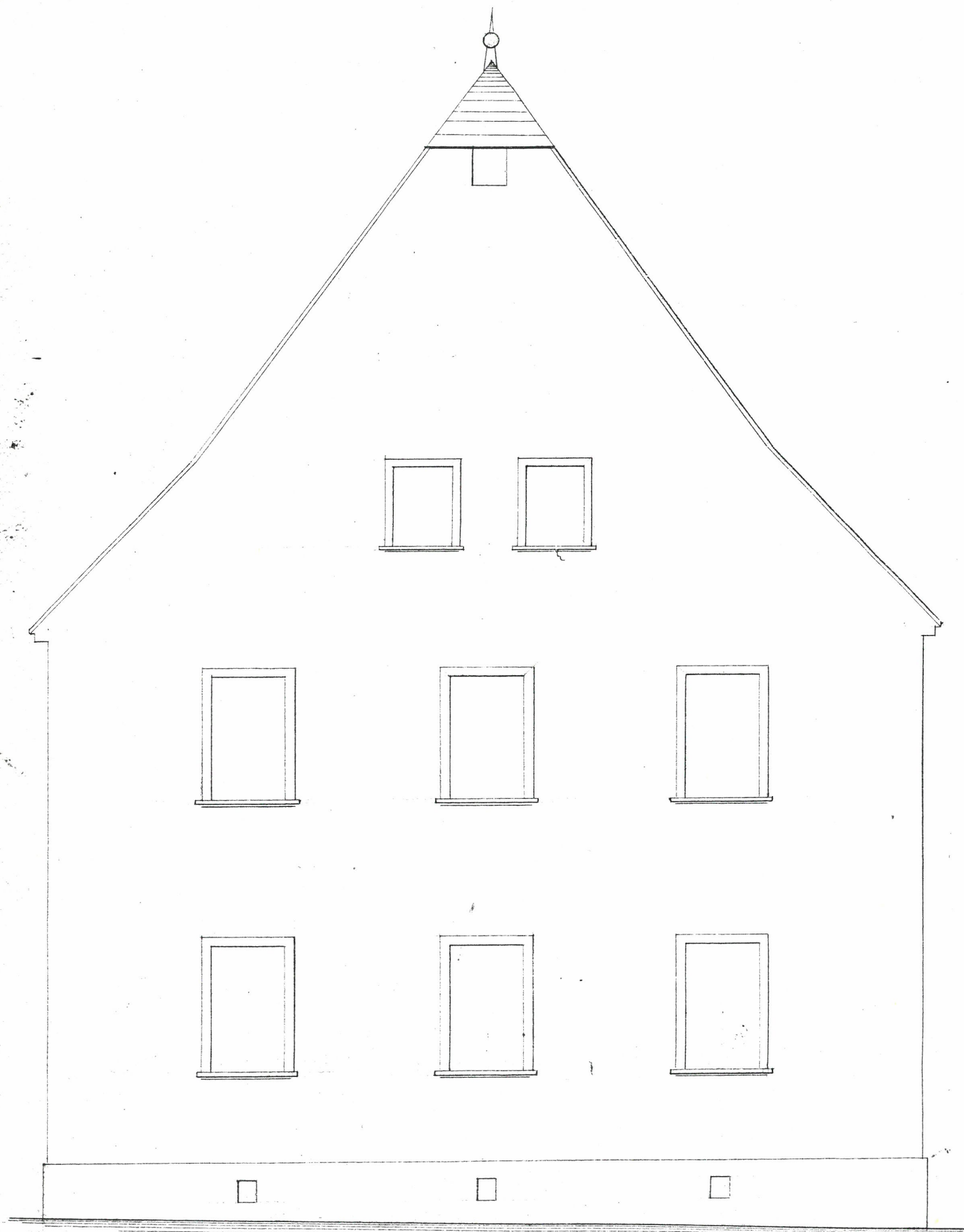
Giebel-Ansicht
