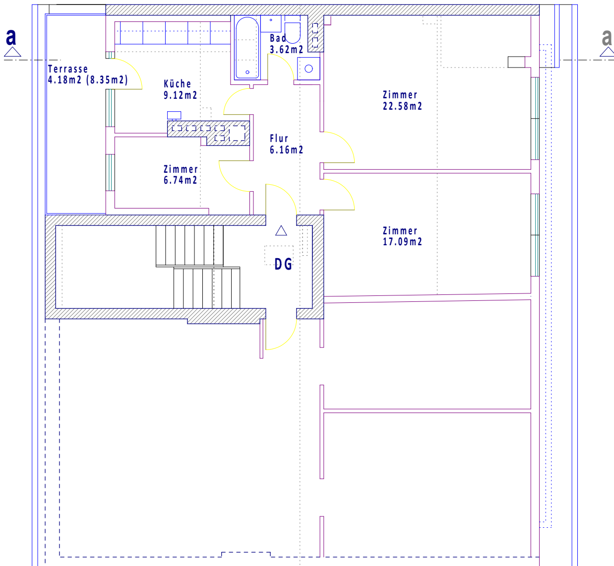
Grundriss
