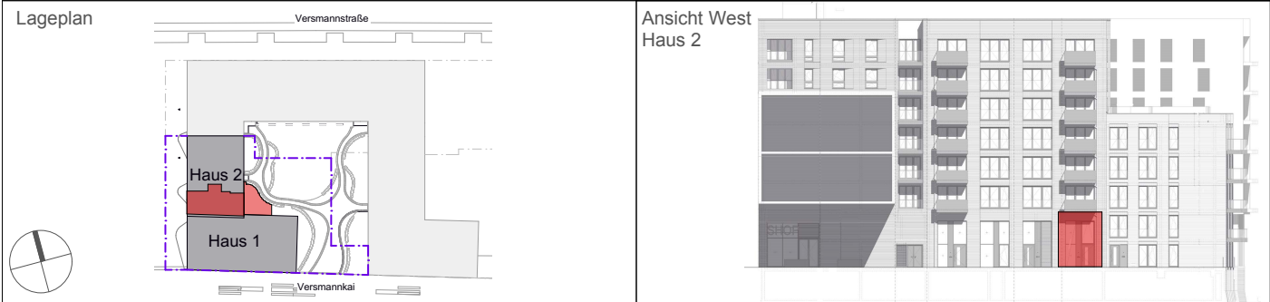
Whg. 2.01 - Erdgeschoss + 1. Obergeschoss (Haus 2) - Maisonette 2 Zimmer - 102,89 m²
