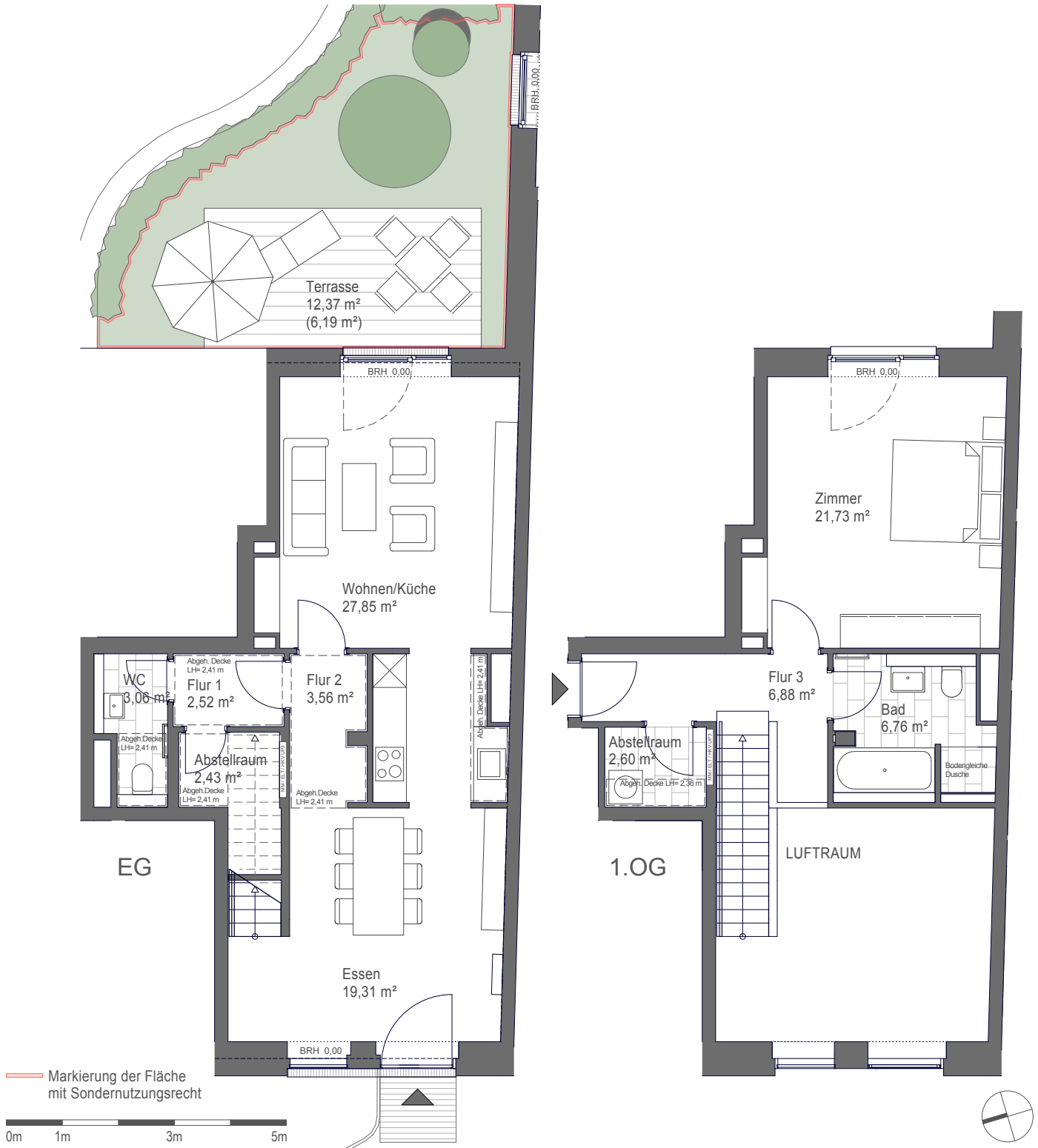
Whg. 2.01 - Erdgeschoss + 1. Obergeschoss (Haus 2) - Maisonette 2 Zimmer - 102,89 m²
