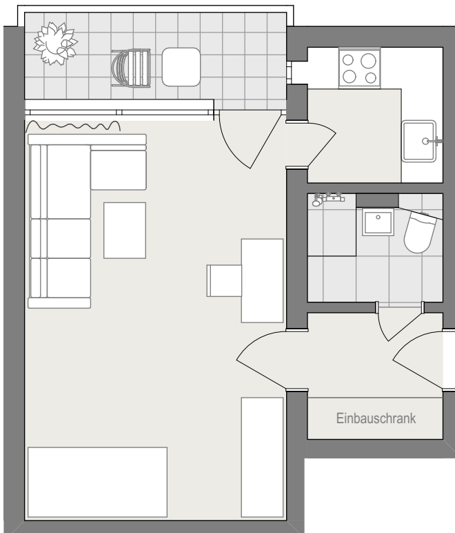
Grundriss Wohnung
