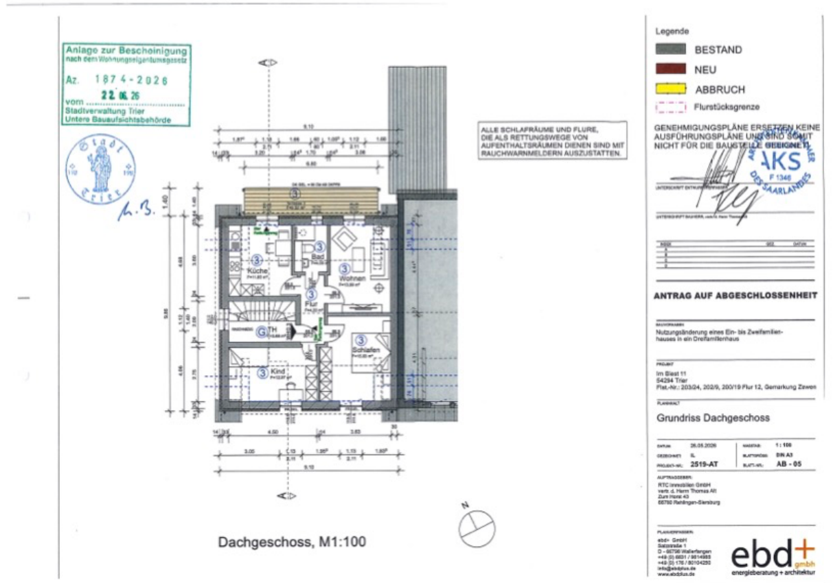
Dachgeschoss, Wohnung 3, mit Raumbezeichnungen und Flächen.
