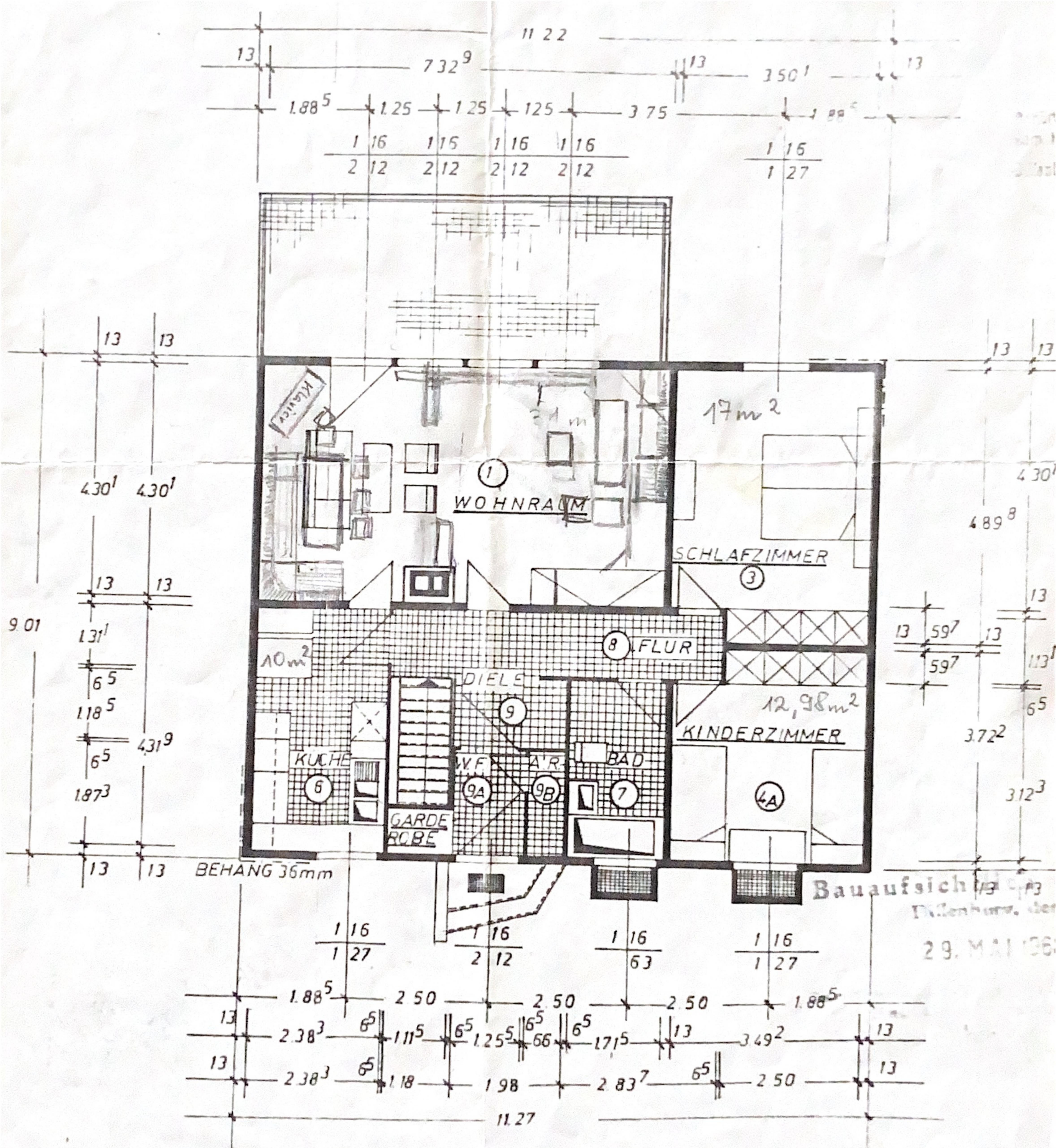
ERDGESCHOSS - GRUNDRISS
