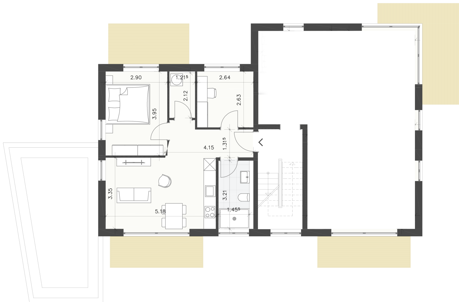
WOHNEINHEIT 4 57m 2 | HAUS 1 | 1.OG
