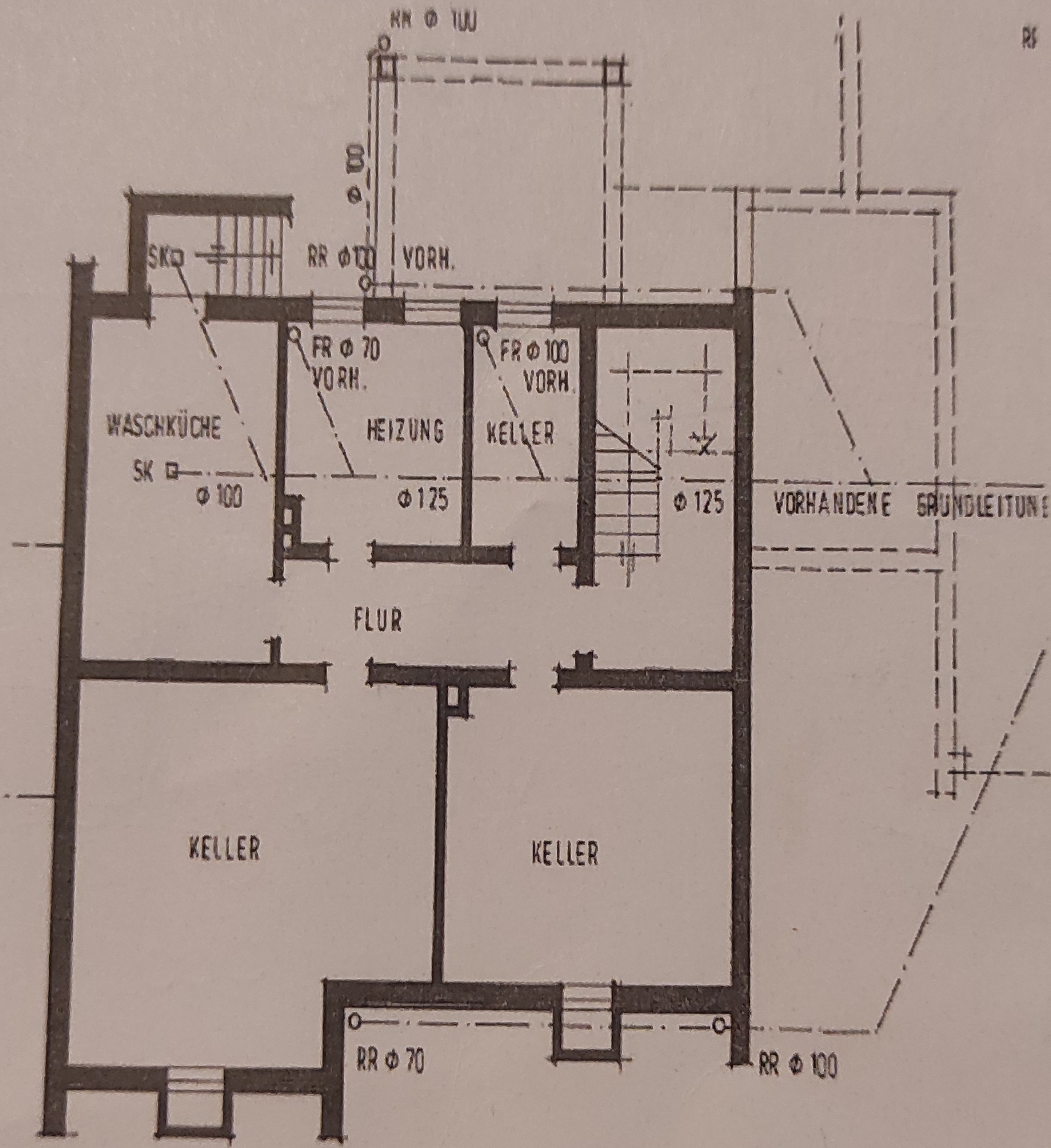
KELLERGESCHOSS
