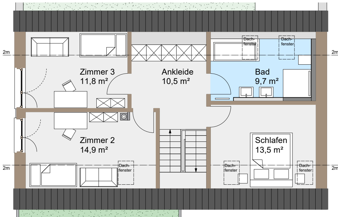
2. Obergeschoss
