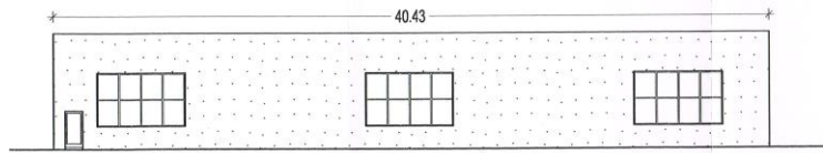
Ansicht Osten
