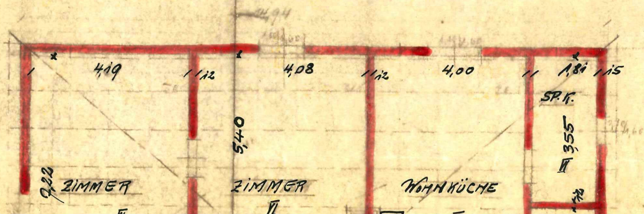
OBERGESCHOSS.
