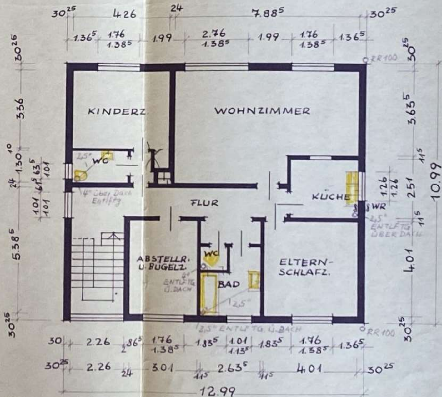
OBERGESCHOSSGRUNDRISS = ERDGESCHOSS
