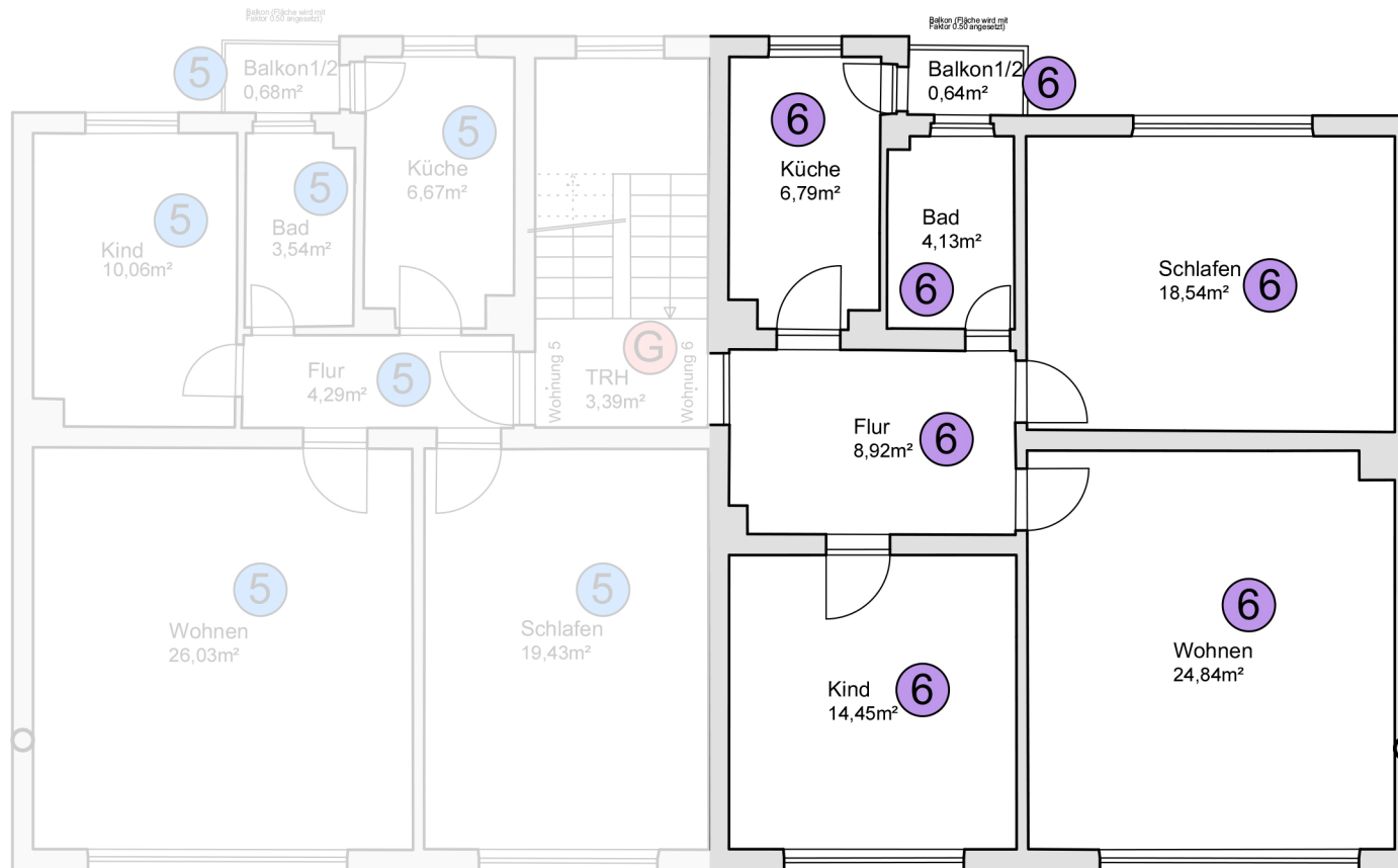
Grundriss 2.Obergeschoss
