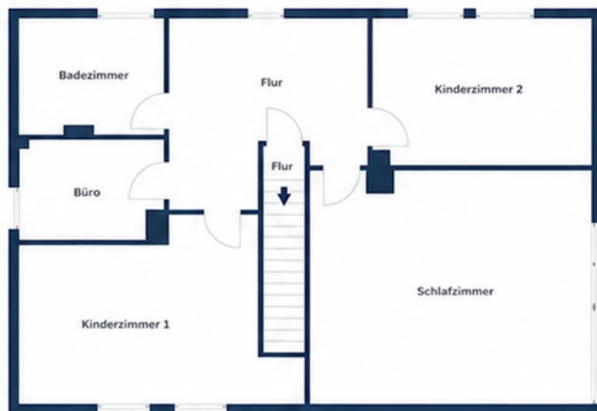
Grundriss 1. OG
