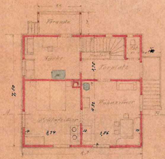
Erstes Geschoss
