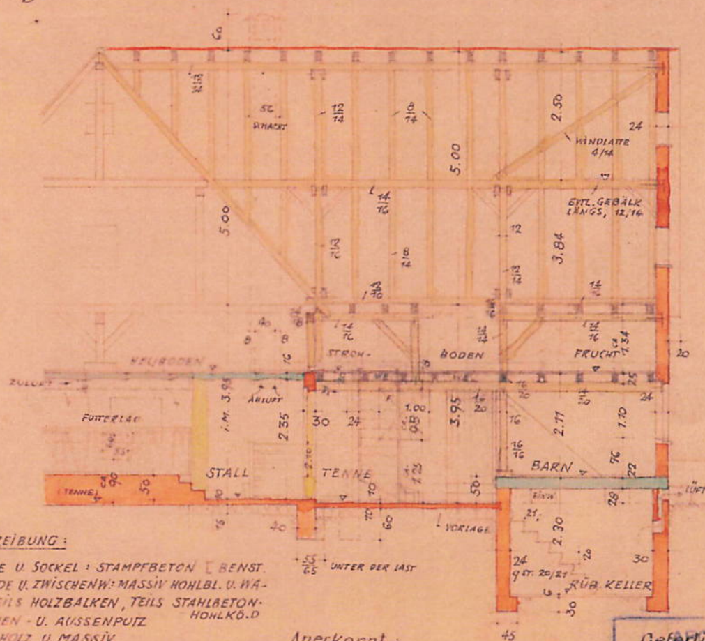
Längsschnitt B-B
