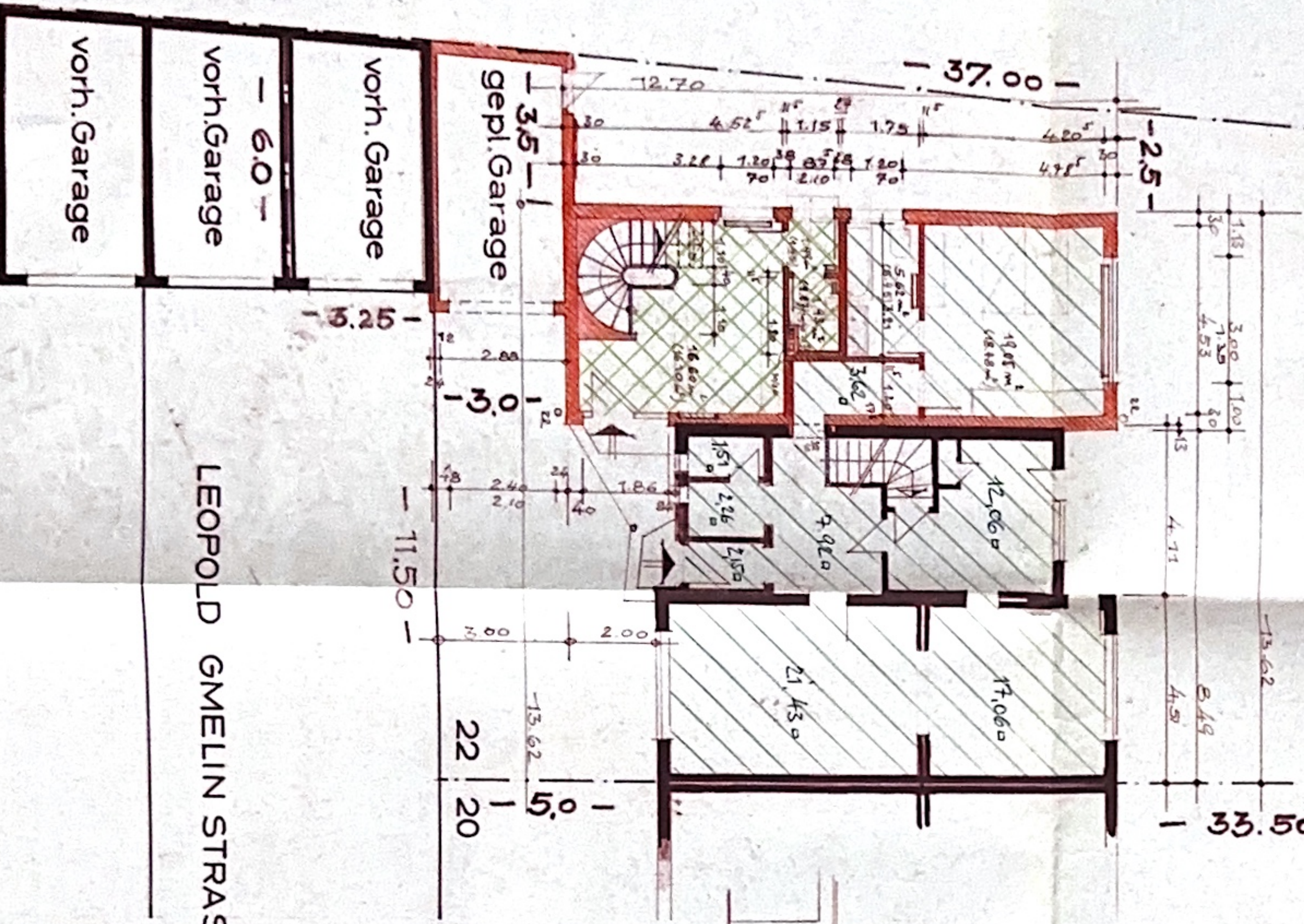
Erdgeschossgrundriss
