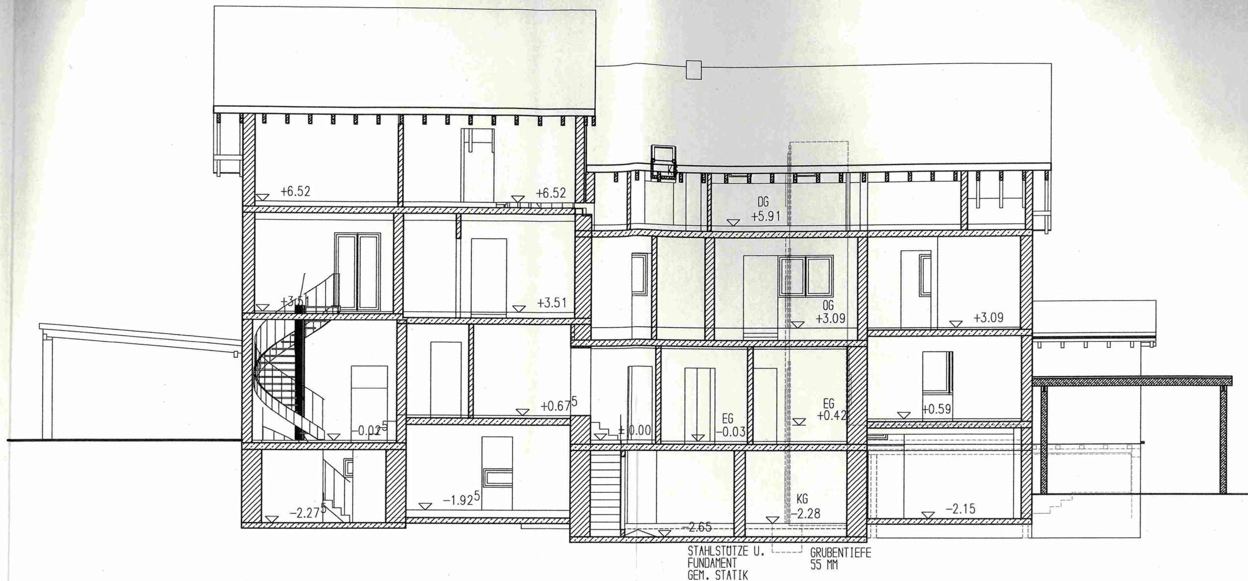
LÄNGSSCHNITT A - A
