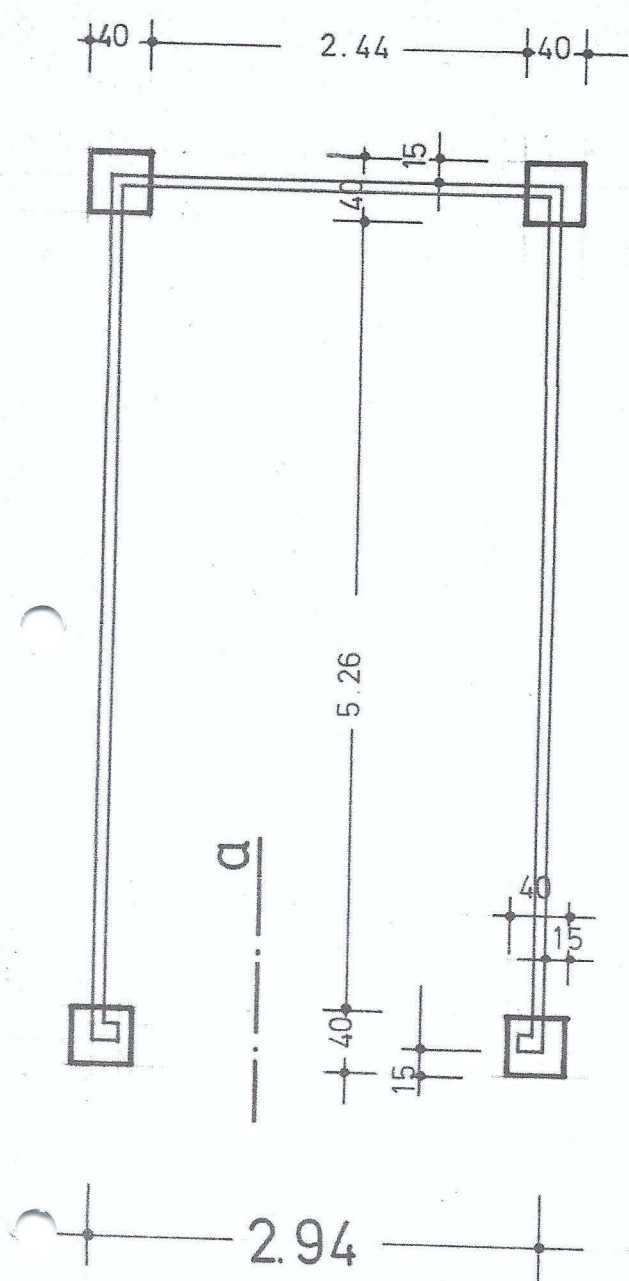
EINZELGARAGE EINZELFUNDAMENT 1:50
