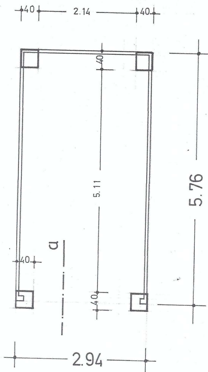
EINZELGARAGE ALS GRENZBAU 1:50
