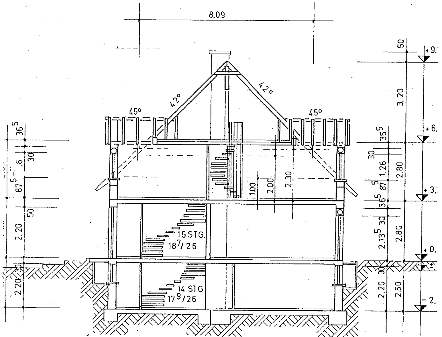
SCHNITT 1
