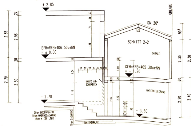
FUNDAMENTE/BODENPLATTE gem. STATIK
