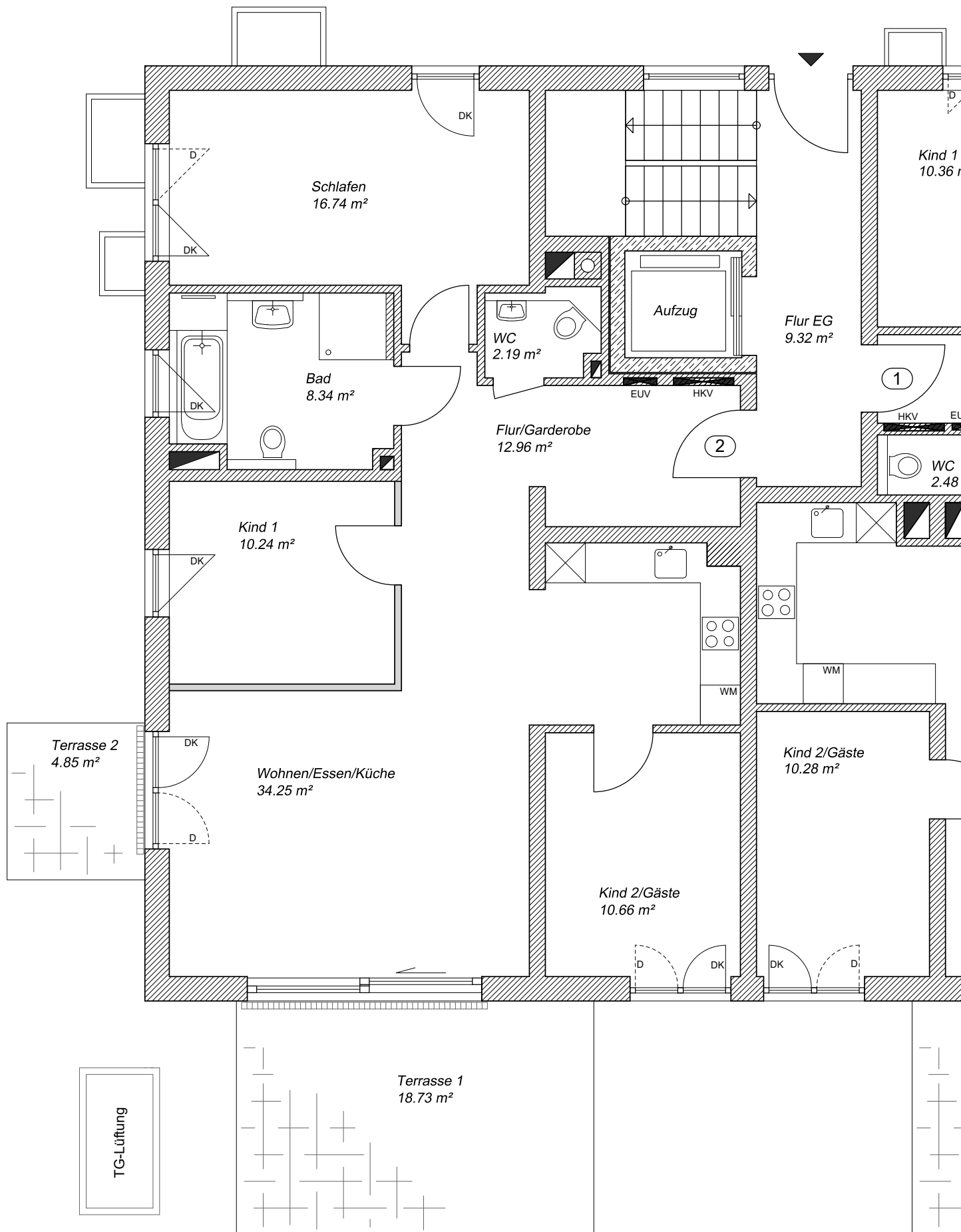
Grundriss Erdgeschoss Wohnung 2
