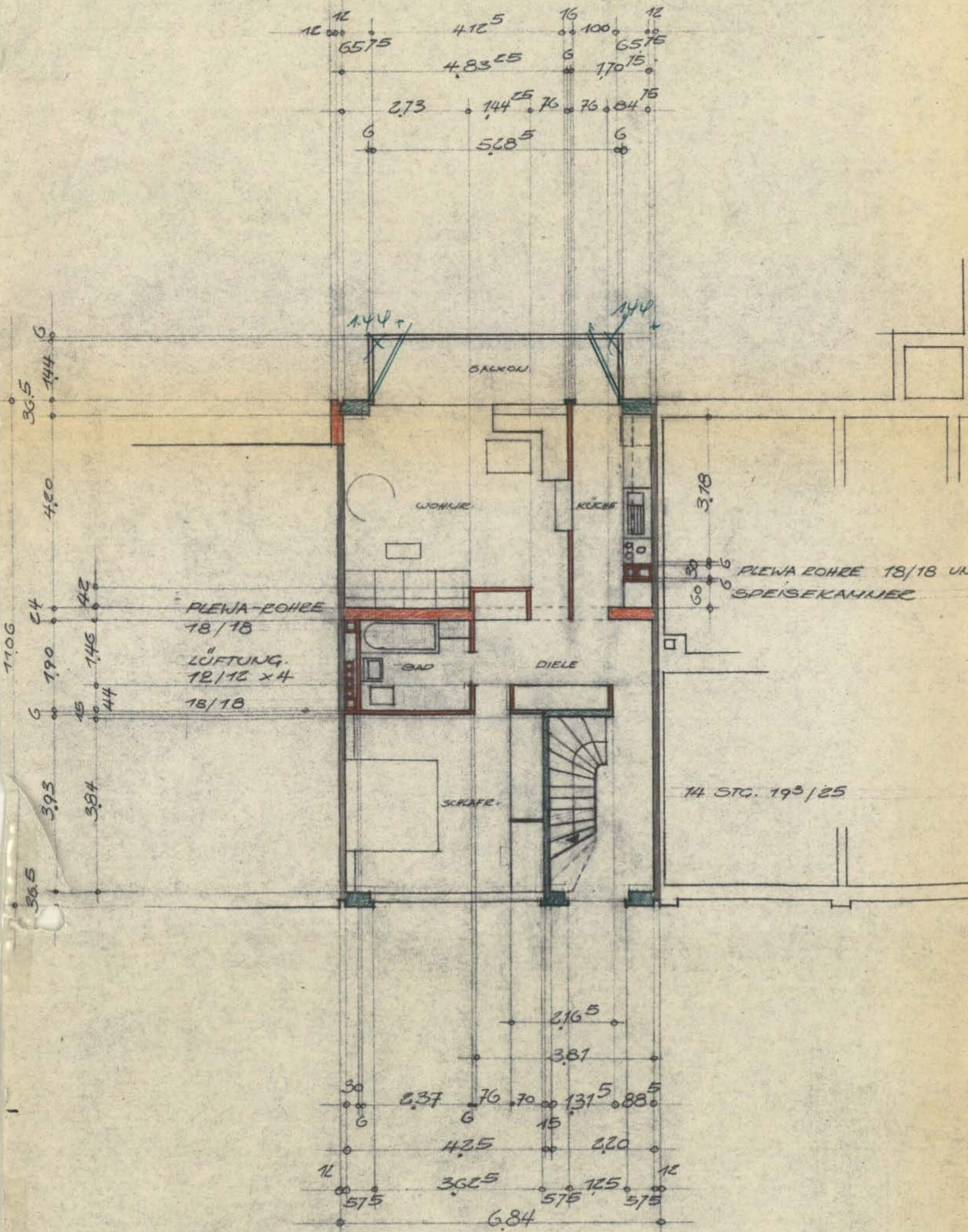
ERD, 1. UND 2. OBERGESCHOSS
