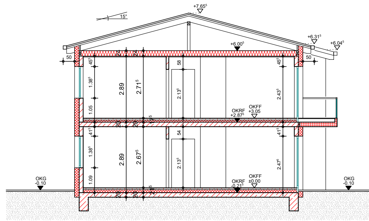
SCHNITT I-I.
