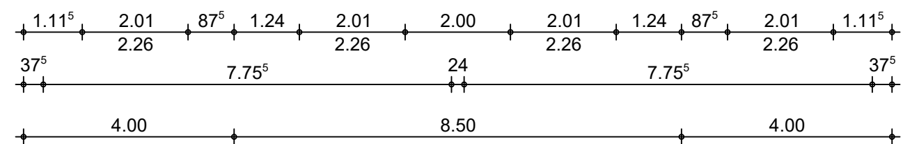
GRUNDRISS EG NF WOHNUNG à 62,88 m² NF ALLGEMEIN 15,43 m²
