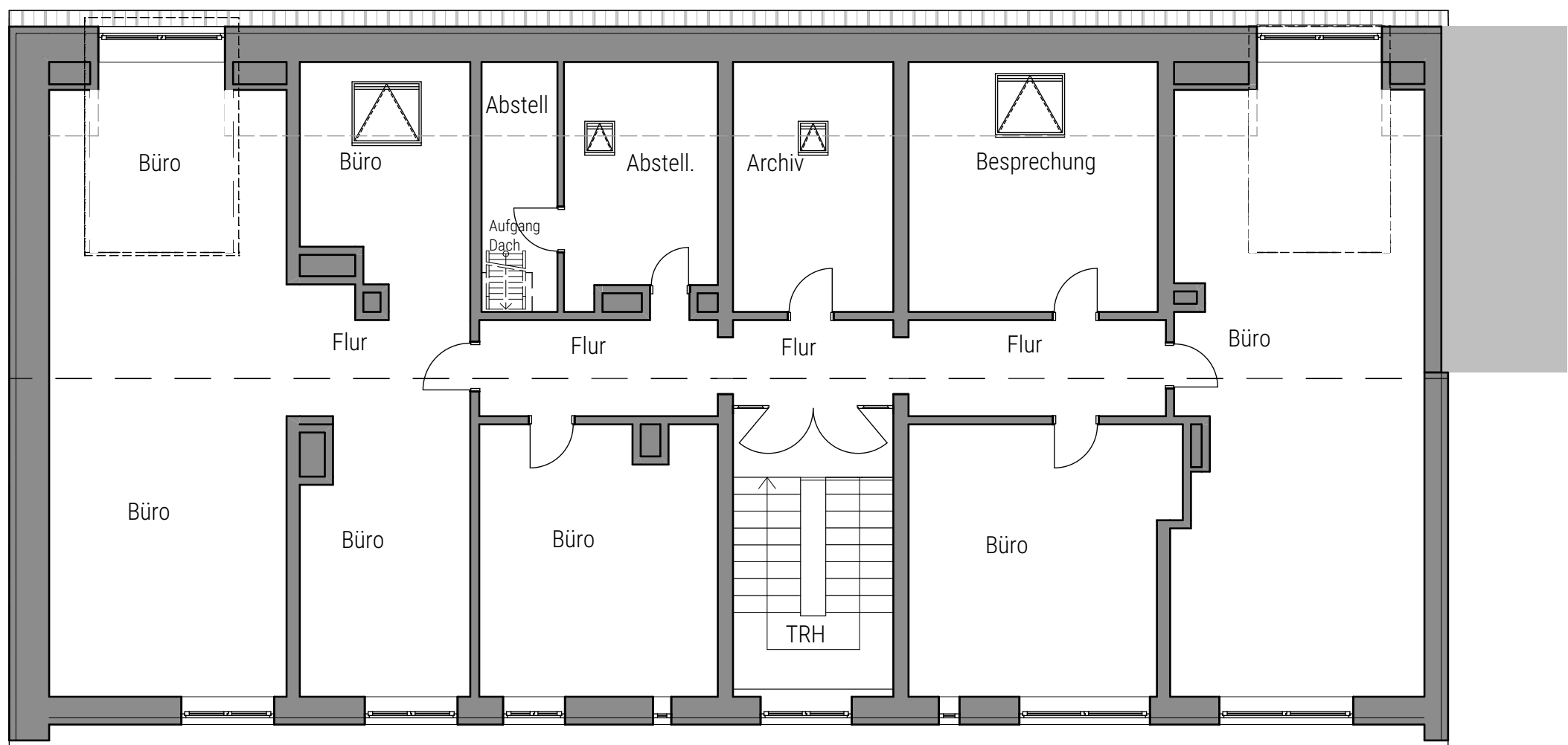
Dachgeschoss
