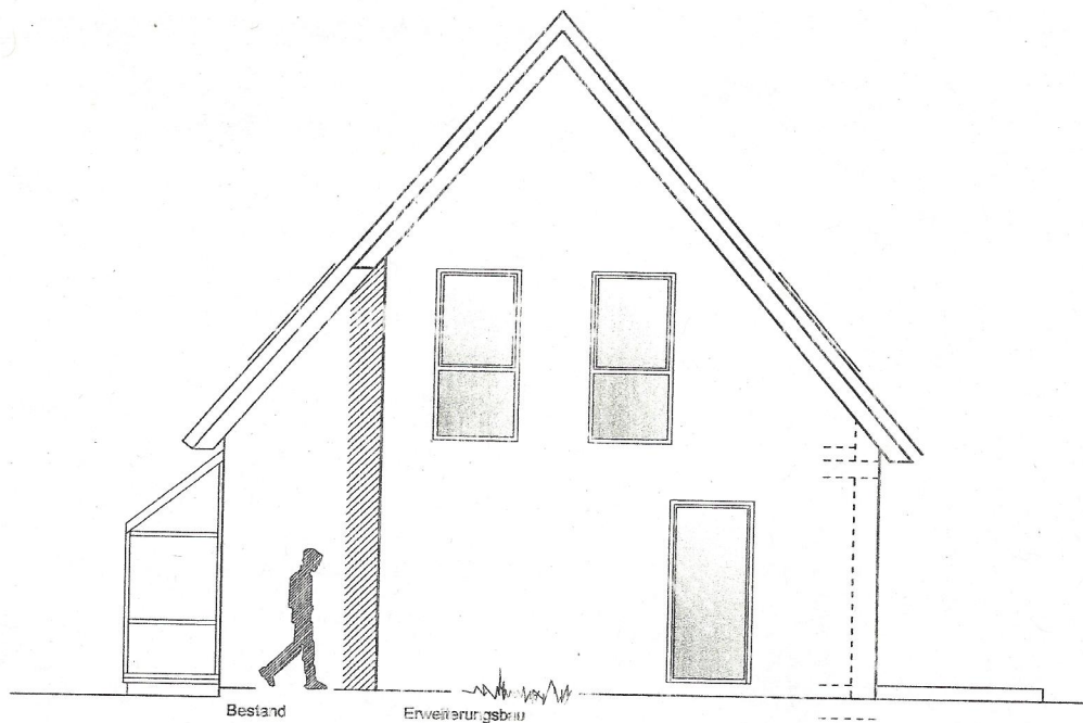
Ansicht Nordost
