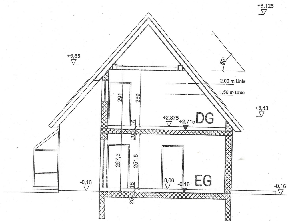
Schnitt B - B (Erweiterungsbau)
